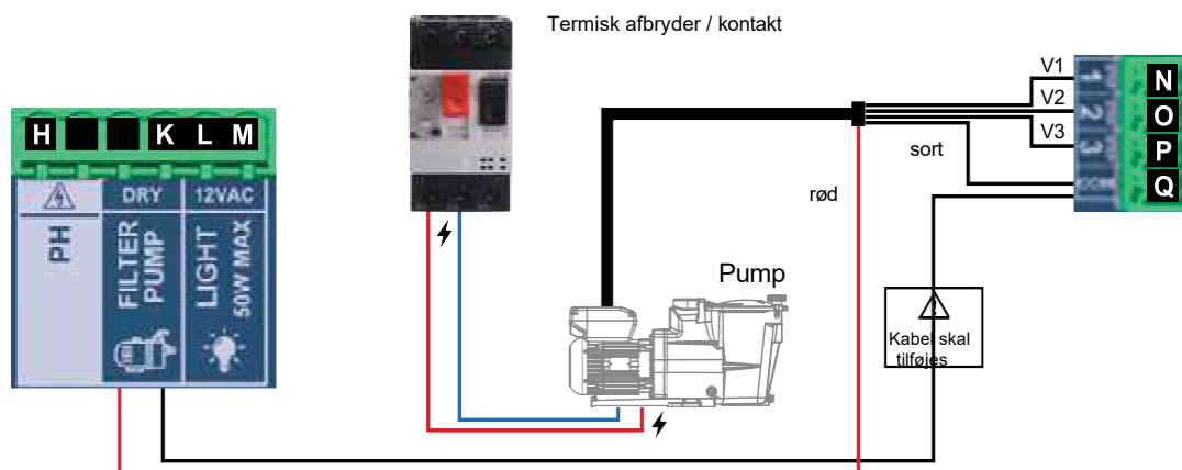
Diagram over installation af pumpe med variabel hastighed på AquaRite® HC LS
