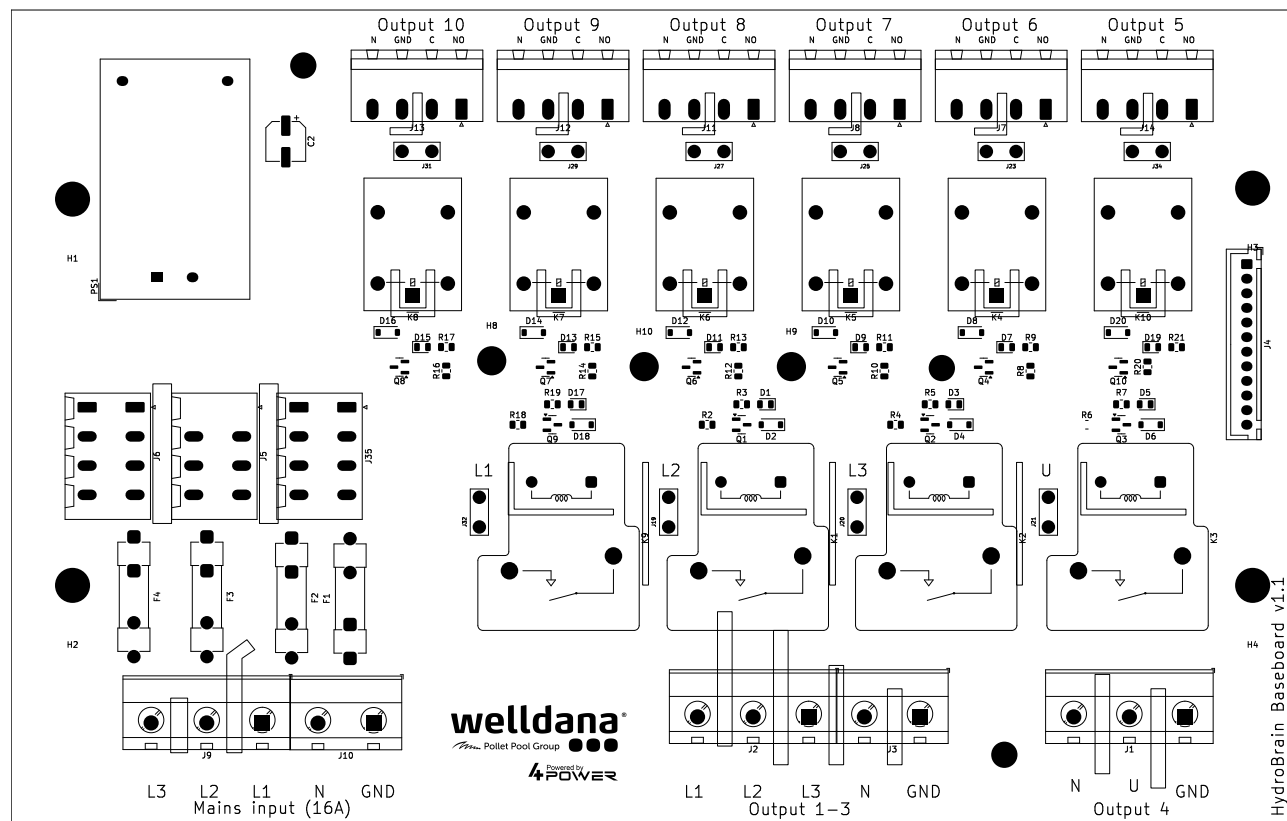
Figur 1: Strømforsyning og effektprint
